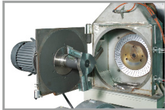
模頭風冷切粒
